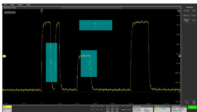
图 3 布尔逻辑触发判定。采用逻辑 OR 的布尔逻辑可以触发信号中的特定异常事件。
