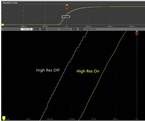
6 系列 MSO 的 12 位 ADC 及新型 High Res 模式实现了业界领先的垂直分辨率。
