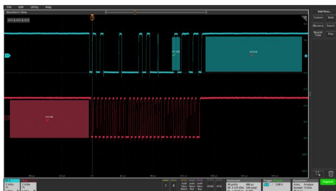
图 2 多条通道触发。可视触发可以与跨越多条通道的事件相关，比如同时在两个总线信号上传送的包。
