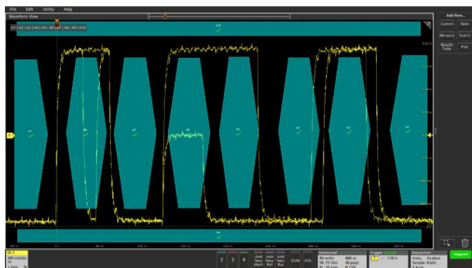
图 1 可视触发区域隔离对应的事件，只捕获要查看的事件，节省时间。
