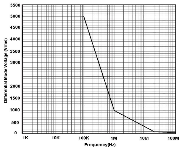
图 4: DP6700B 最大差模电压 VS 频率
