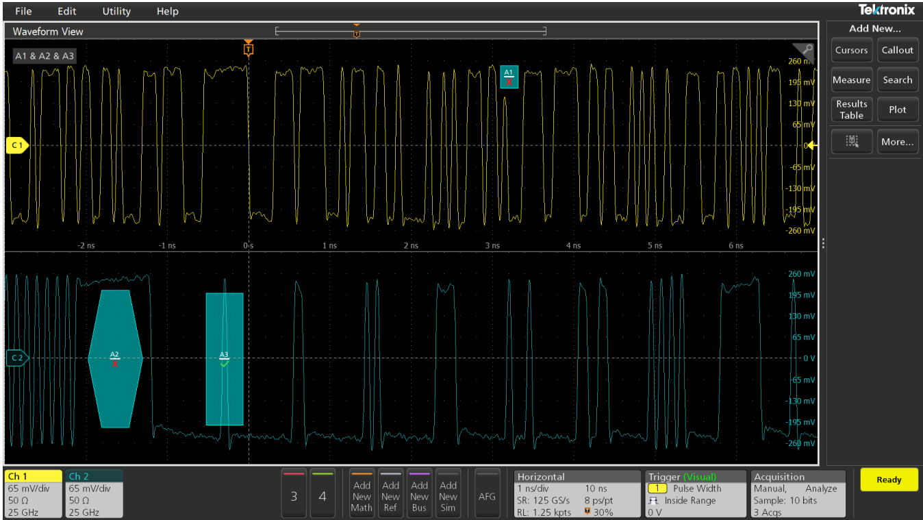
多条通道触发。可视触发可以与跨越多条通道的事件相关，比如同时在两个总线信号上传送的数据包。
