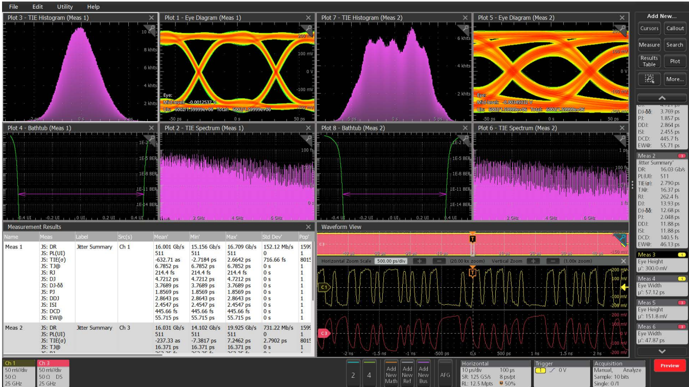
多路信号抖动与眼图的并行比较。
