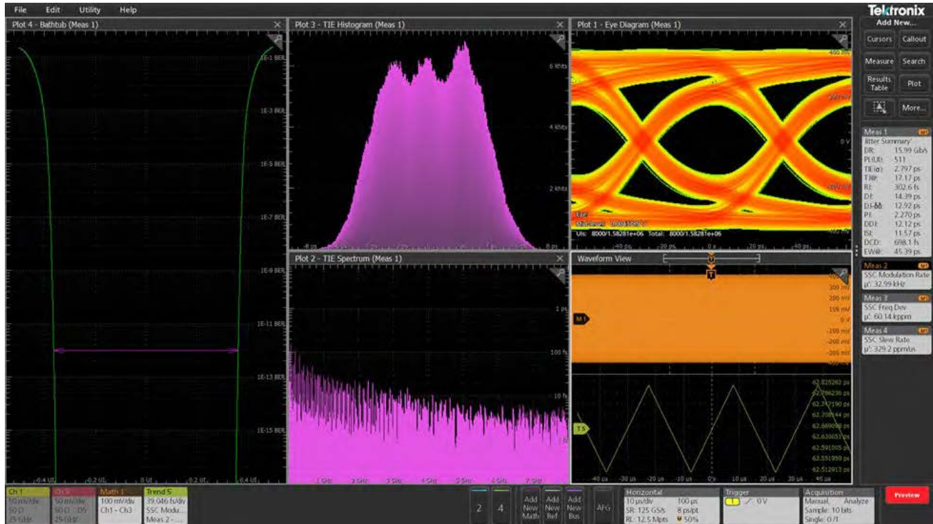
“抖动摘要”结合展频时钟 (SSC) 测量，可在数秒内全面呈现设备的性能表现。
