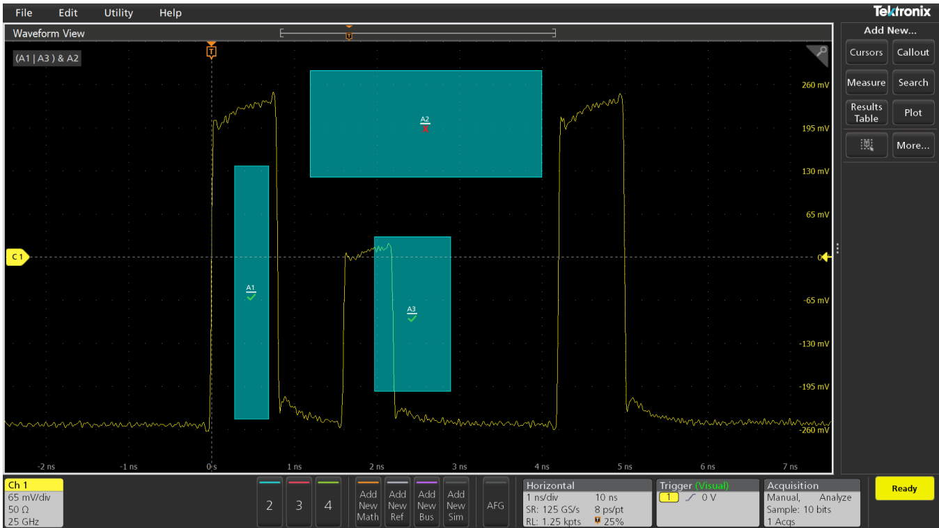
布尔逻辑触发判定。采用逻辑OR的布尔逻辑可以触发信号中的特定异常事件。
