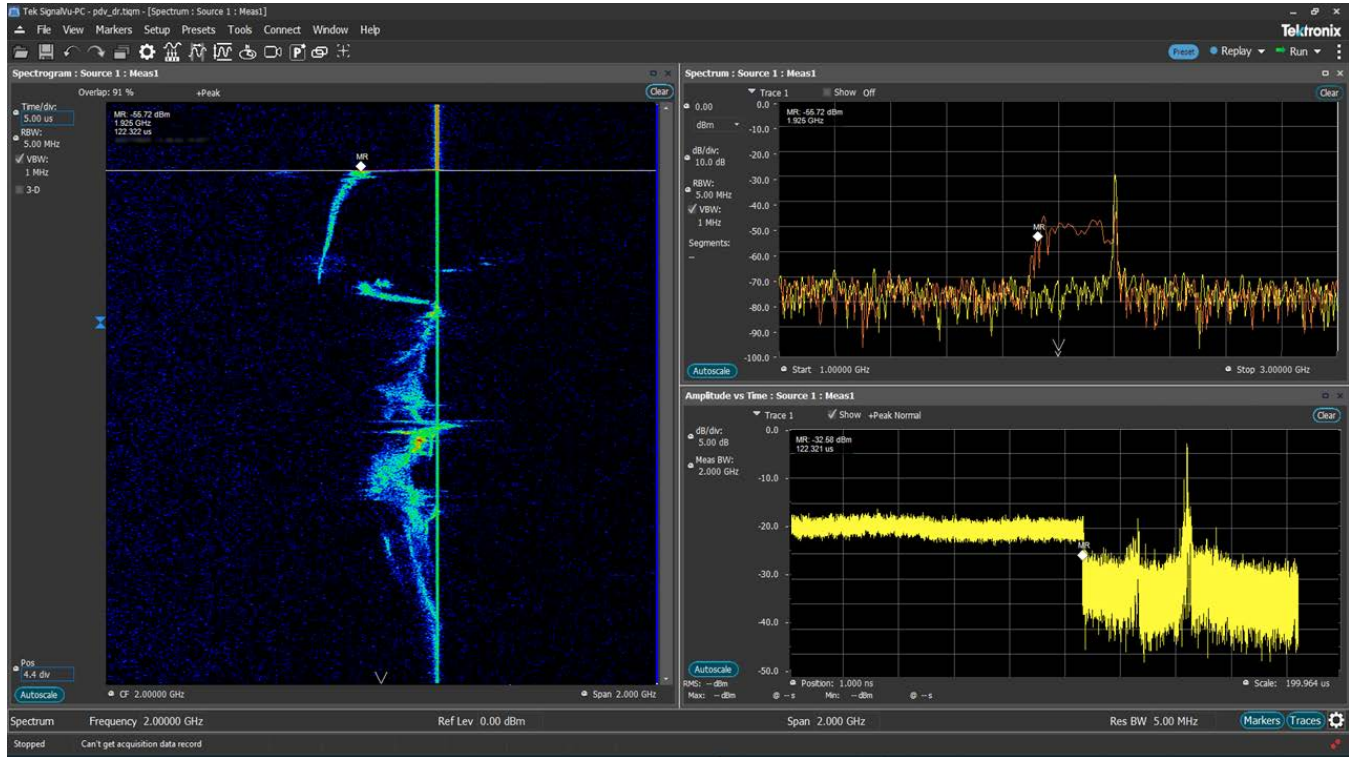
使用SignalVu-PC的频谱图显示功能快速呈现快速事件，现已支持深色模式。
