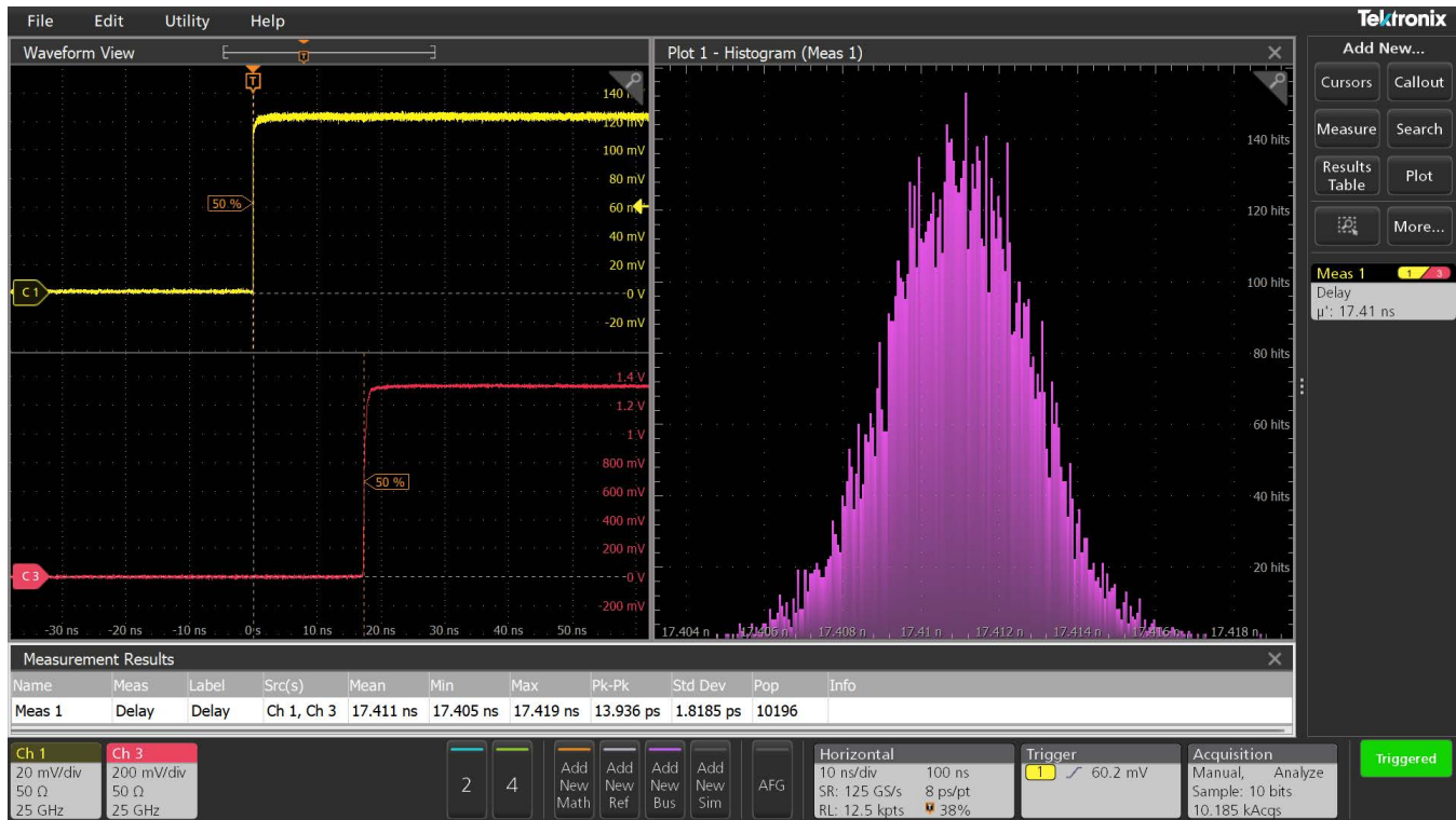
通道 1 至辅助输出的触发延迟测量值 < 20 ns。
